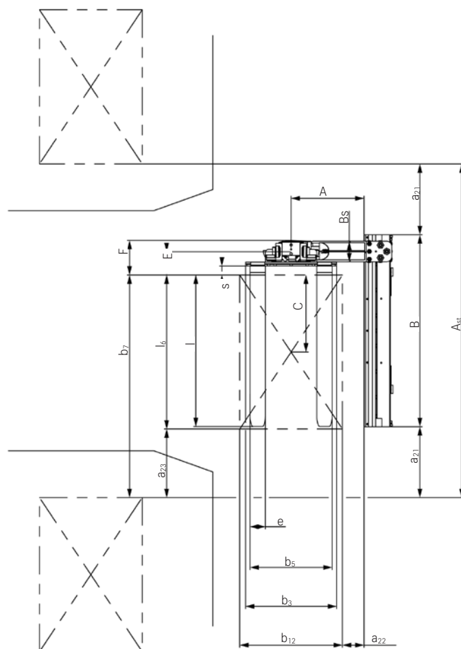
Otočná výsuvná vidlice – pohled shora
